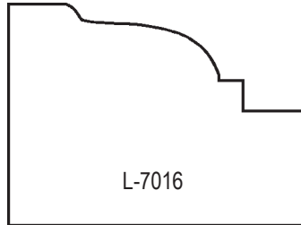
CORNICE MOLD 1-1/4 X 1-3/4 V.G. FIR
